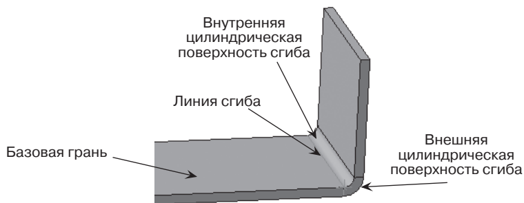
Рис. 365. Элементы листового тела
