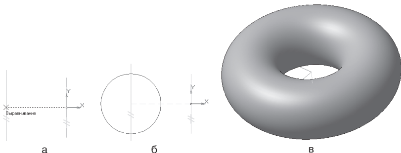
Рис. 137. Создание трехмерной модели тора
