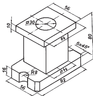
б) Опора.
