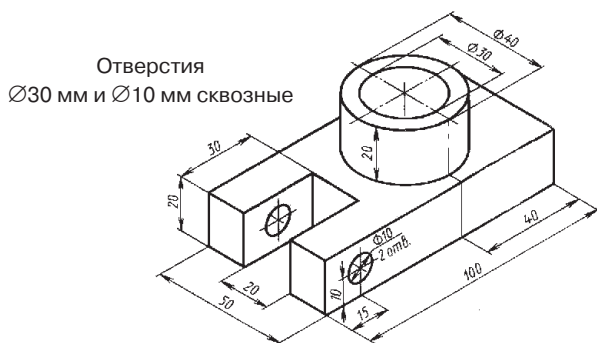
Рис. 293. Направляющая
