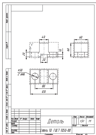
Рис. 2. Объемная модель с соответствующим чертежом
