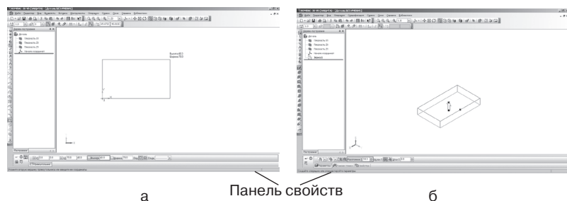
Рис. 116. Панель свойств
