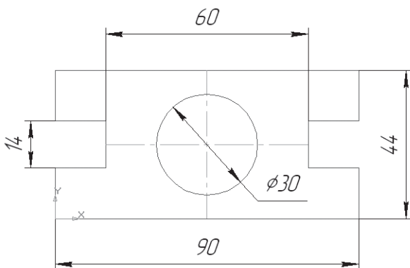
Рис. 33. Чертеж пластины
