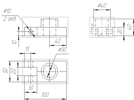
Рис. 354. Чертеж с простановкой размеров
