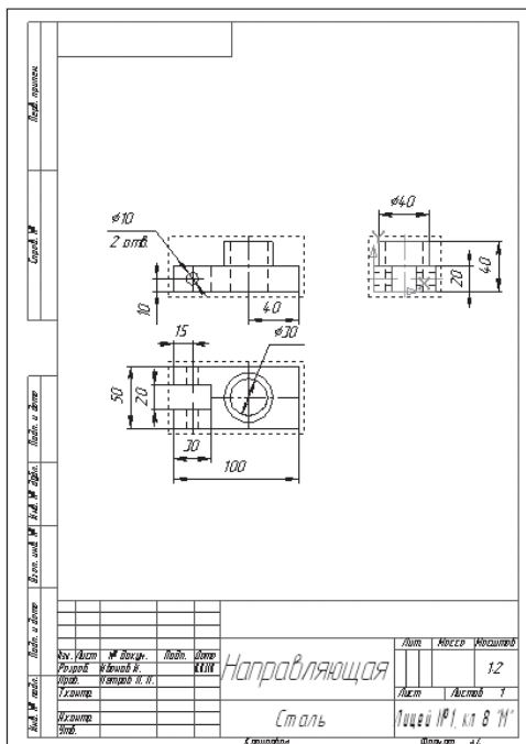
Рис. 360. Направляющая
