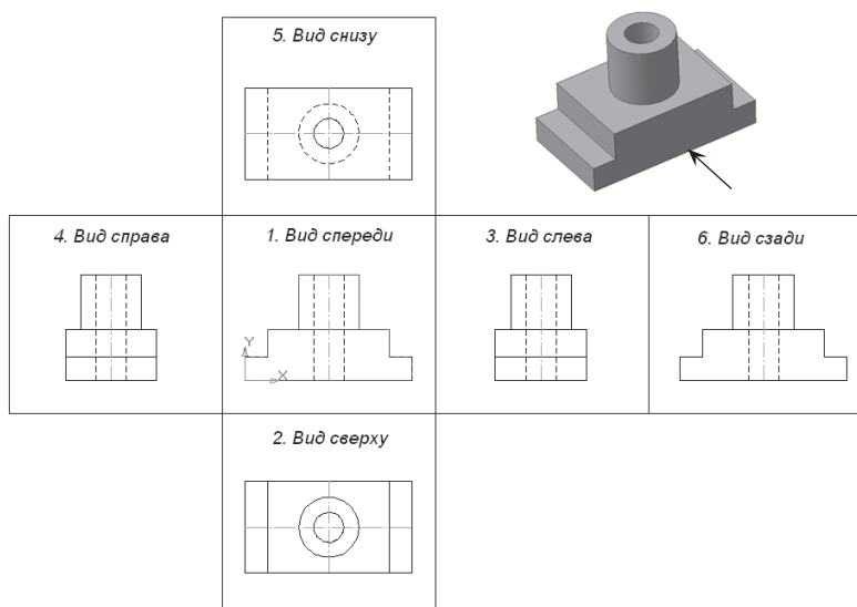
Рис. 292. Расположение видов на чертеже относительно главного вида
