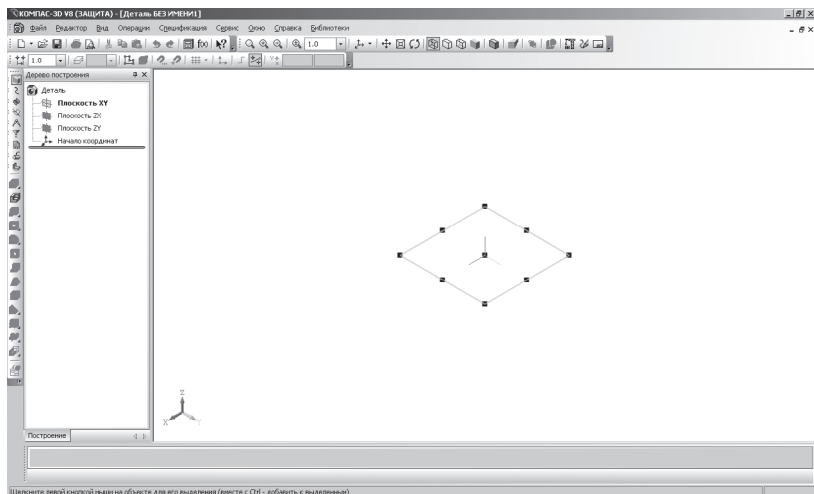
Рис. 121. Выбор плоскости
