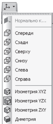
Рис. 113. Ориентация
