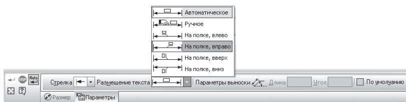
Рис. 346. Вкладка Параметры
