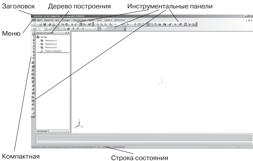
Рис. 111. Окно документа
