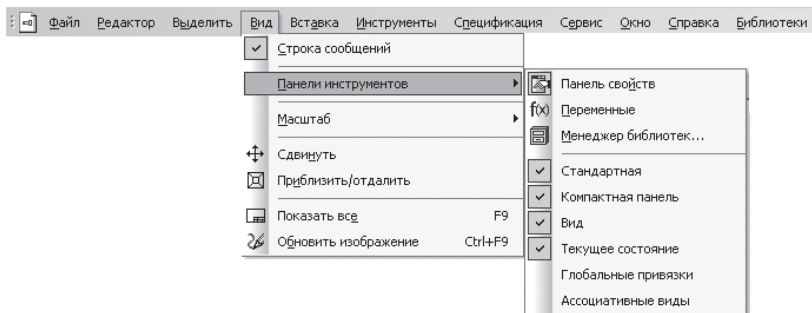
Рис. 12. Главное меню
